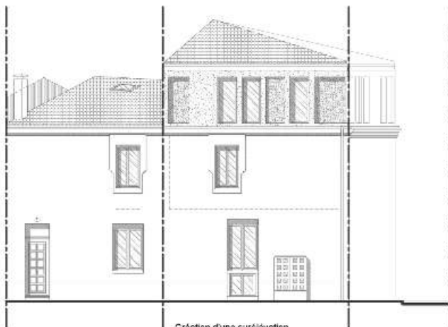
Création d'une surélévation & modifications de façades & ravalement
