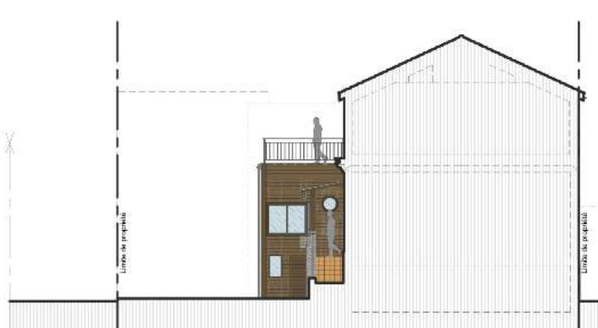
Maison de village Coupe - projet Construction d'une surélévation & Modification de façade
