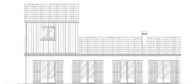
Création d'une surélévation
