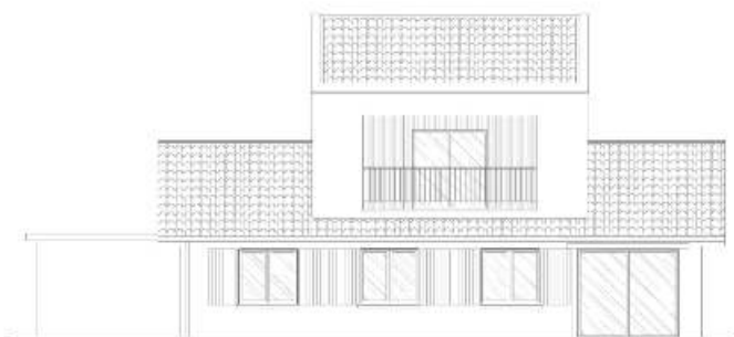
Création d'une surélévation
