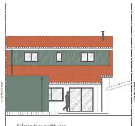
Création d'une surélévation par prolongement de toiture
