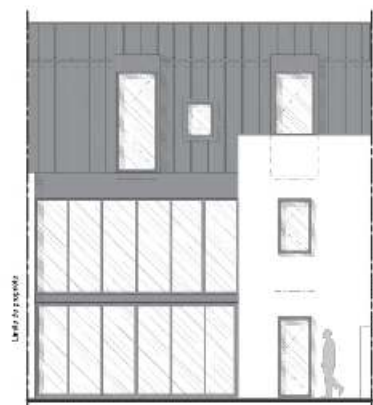
Création d'une surélévation & extension & modifications de façades
