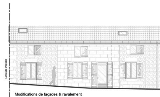
Modifications de façades & ravalement
