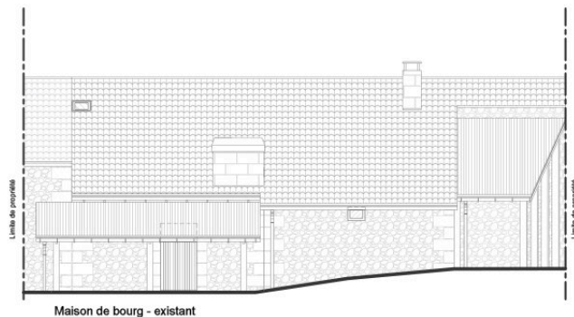
Maison de bourg - existant
