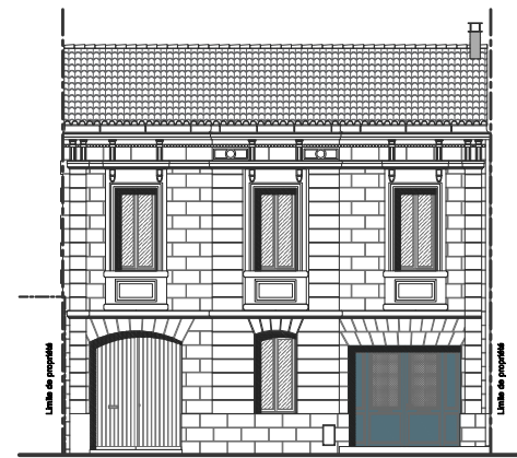
Maison de ville - existant / travaux de ravalement & remplacement Mext.
