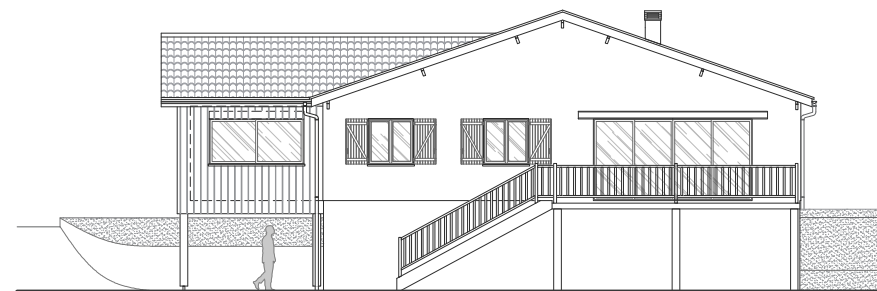
Création d'une extension sur pilotis
