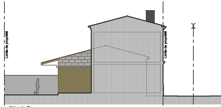
Maison de ville Coupe longitudinale - existant
