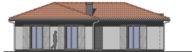
Maison Individuelle Façade sur rue - Modification de façade (Ravalement)
