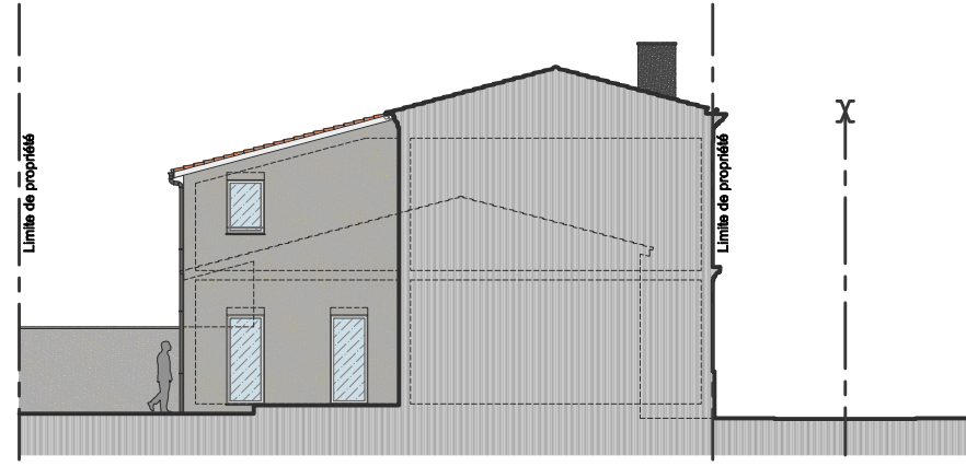
Maison de ville Coupe longitudinale - Extension
