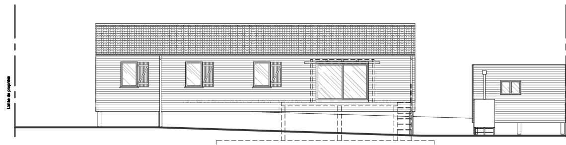
Création d'une extension
